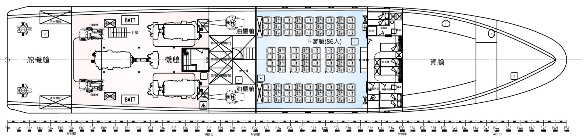
下甲板客艙
